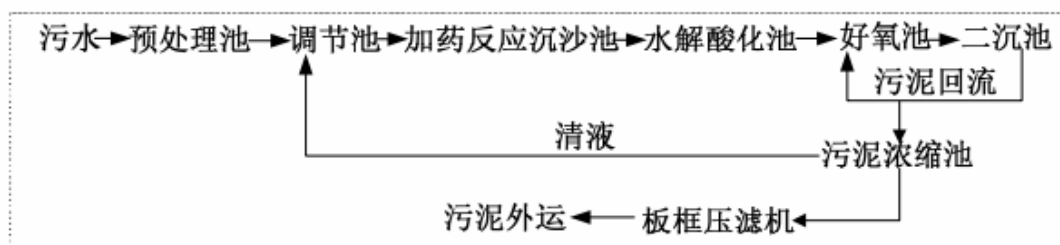
图 2-1 污水处理工艺流程
